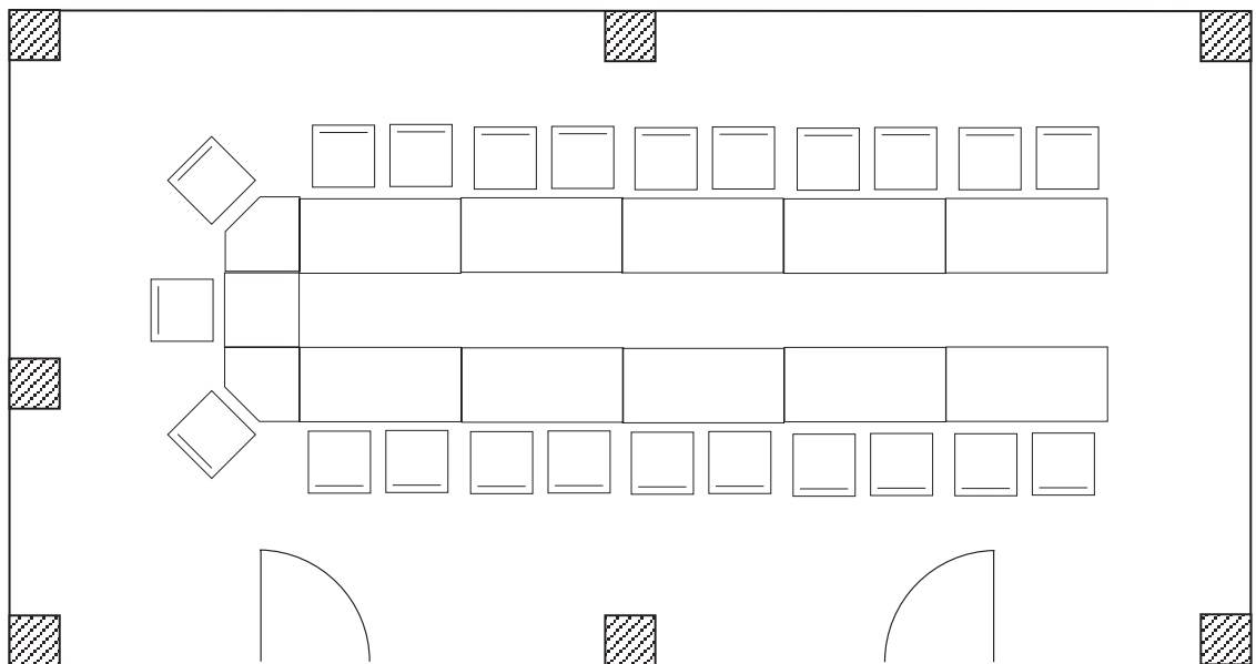
Beispiel »B2« für 23 Personen
